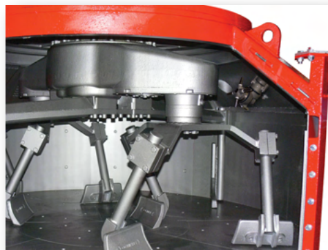
Tête A80R installée dans la couverture d'accès du mélangeur planétaire
